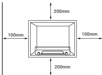
Casete șemineu
